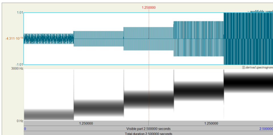
Fig. 2 Representación gráfica de la forma de onda de la secuencia 2
